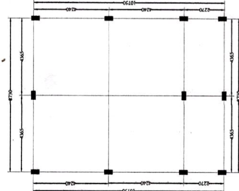
COLUMN LAYOUT PLAN SCALE: 1: 100
